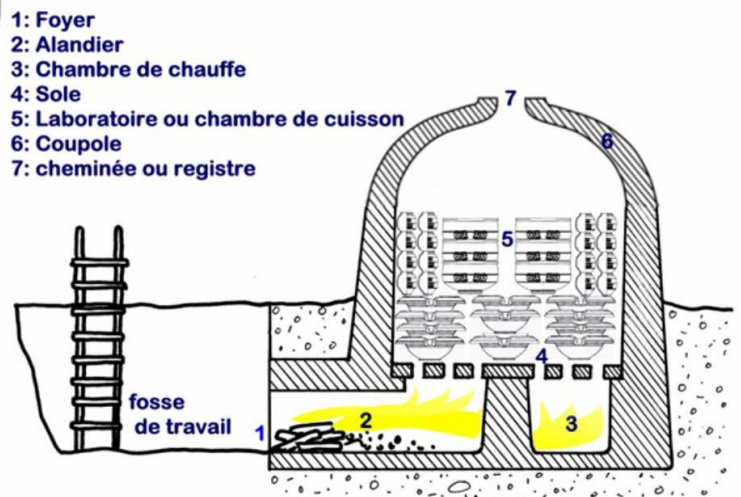
Schéma d'un four de potier
